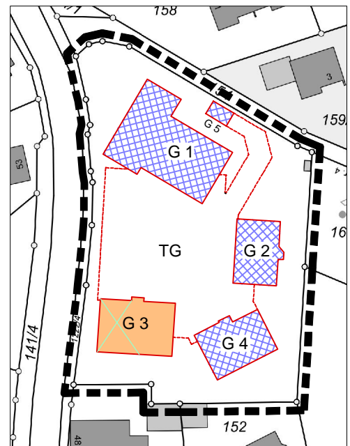
ÜBERSICHTSPLAN
