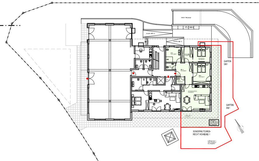
ÜBERSICHTSPLAN ERDGESCHOSS
